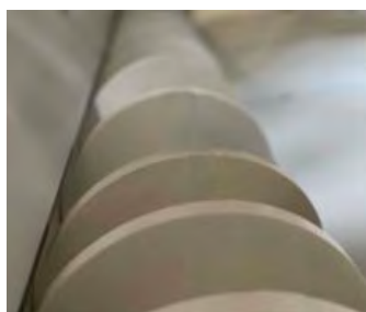
Extraction par vis sans fin à pas variable en matière plastique alimentaire
